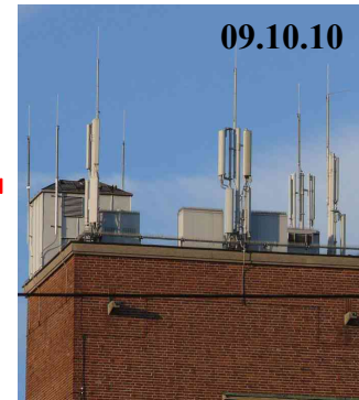
Mobilfunksendeanlage Eichamt Montagehöhe: 34-36 m 30 Sektorantennen (Stand 2009) Erstinbetriebnahme 1999
